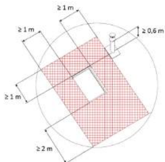
A - B Dachfenster
