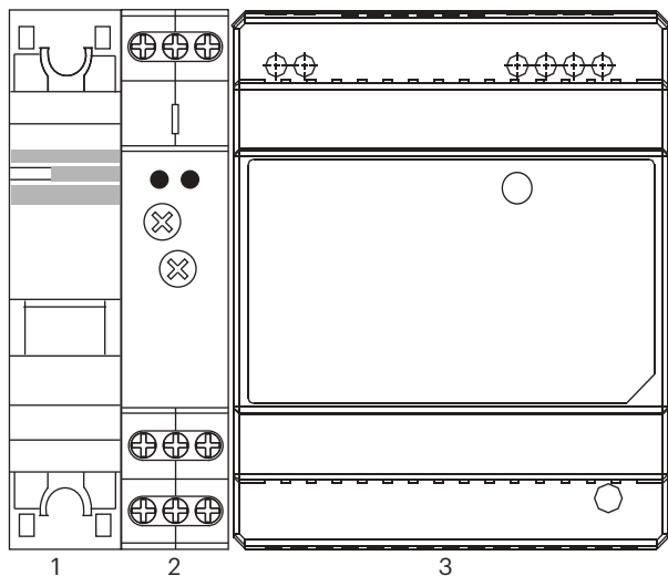
1- выключатель; 2- реле задержки выключения; 3- блок питания
