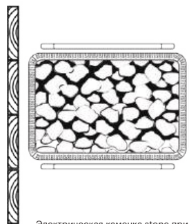
Электрическая каменка stone прилегает к стене одной стороной
