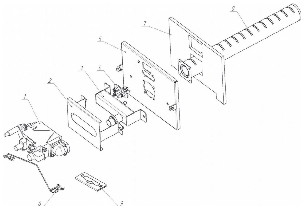
Рисунок 7 -Монтаж газогорелочного устройства
