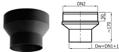
RD x/y - CZ 2/II - S
