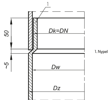
Rys. Sposób łączenia elementów przyłączy kominowych SPK
