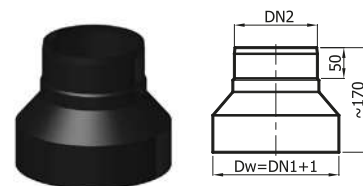
RD x/y - CZ 2/I - S
