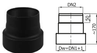
RD x/y - CZ 2/I
