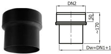
RD x/y - CZ 2/II
